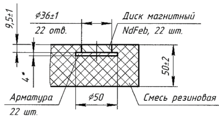
A-A(1:2,5)
